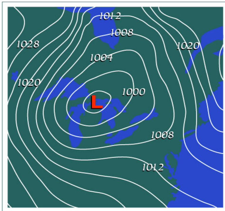
Σχήμα 1 : Βαρομετρικό χαμηλό με κέντρο 996 hPa (πηγή: www.newmediastudio.org )
