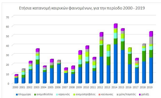
Σχήμα 10. Ετήσια κατανομή καιρικών φαινομένων, για την περίοδο 2000 - 2019
