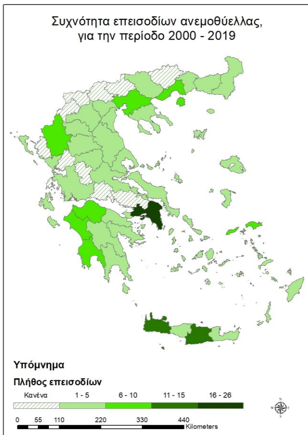
Σχήμα 15. Συχνότητα επεισοδίων ανεμοθύελλας με κοινωνικές και οικονομικές επιπτώσεις ανά νομό, για την περίοδο 2000 – 2019.
