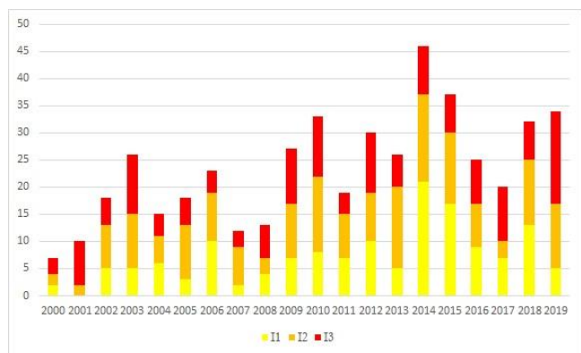
Σχήμα 3. Ετήσια κατανομή αριθμού επεισοδίων ανά ένταση επιπτώσεων, για την περίοδο 2000 - 2019
