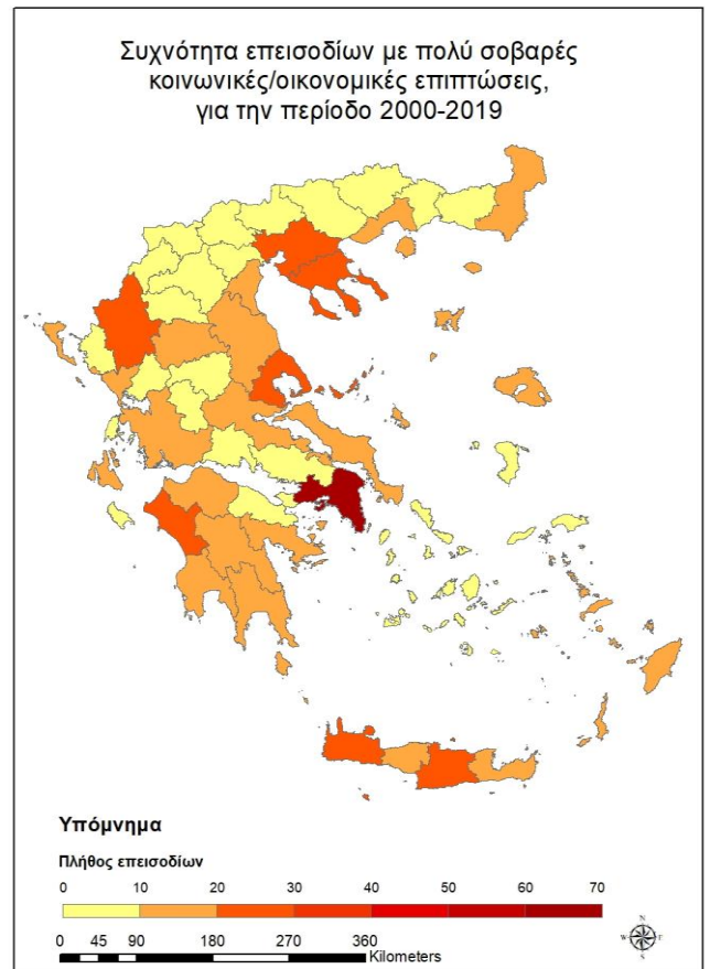
Σχήμα 12. Συχνότητα επεισοδίων ανά νομό, με πολύ σοβαρές κοινωνικές/οικονομικές επιπτώσεις, για την περίοδο 2000 - 2019.
