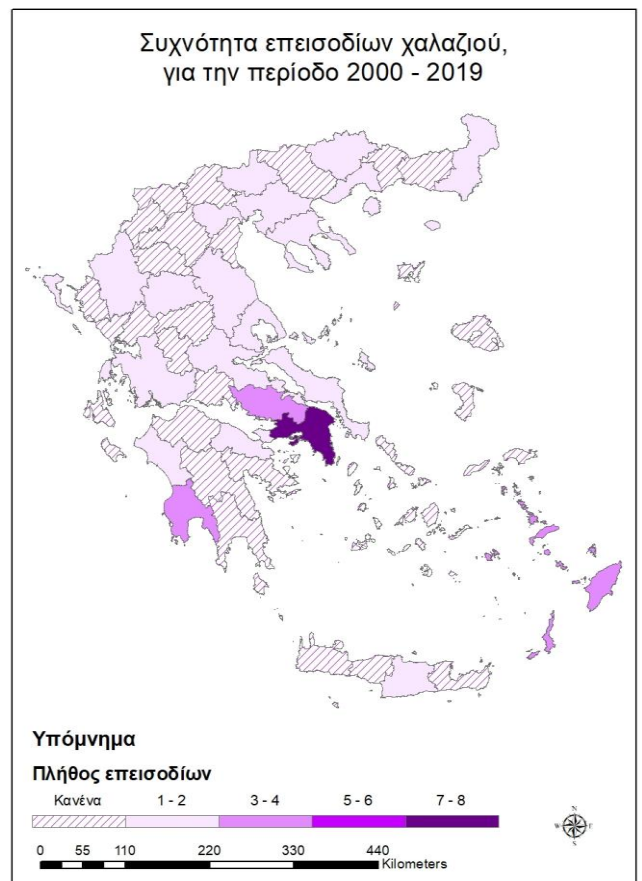
Σχήμα 19. Συχνότητα επεισοδίων χαλαζιού με κοινωνικές και οικονομικές επιπτώσεις ανά νομό, για την περίοδο 2000 – 2019.
