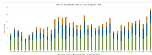
Σχήμα 2. Ετήσια κατανομή καιρικών φαινομένων με οικονομικές απώλειες στην Ευρώπη, για την περίοδο 1980-2018 (πράσινο: μετεωρολογικά, μπλε: υδρολογικά, πορτοκαλί: κλιματολογικά). Πηγή: Munich Re, 2020
