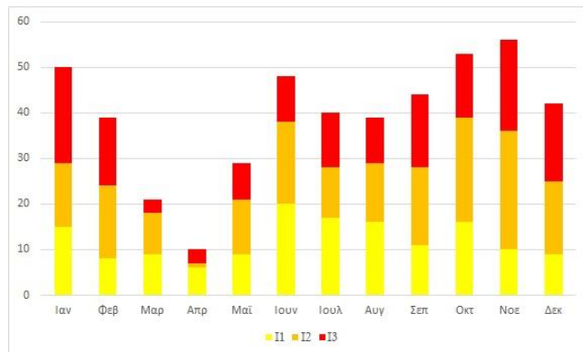
Σχήμα 4. Μηνιαία κατανομή αριθμού επεισοδίων ανά ένταση επιπτώσεων, για την περίοδο 2000 - 2019
