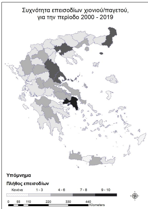
Σχήμα 17. Συχνότητα επεισοδίων χιονιού/παγετού με κοινωνικές και οικονομικές επιπτώσεις ανά νομό, για την περίοδο 2000 – 2019.
