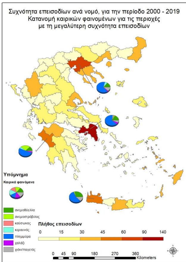
Σχήμα 11. Συχνότητα επεισοδίων ανά νομό, για την περίοδο 2000 - 2019. Κατανομή καιρικών φαινομένων για τις περιοχές με τη μεγαλύτερη συχνότητα επεισοδίων.
