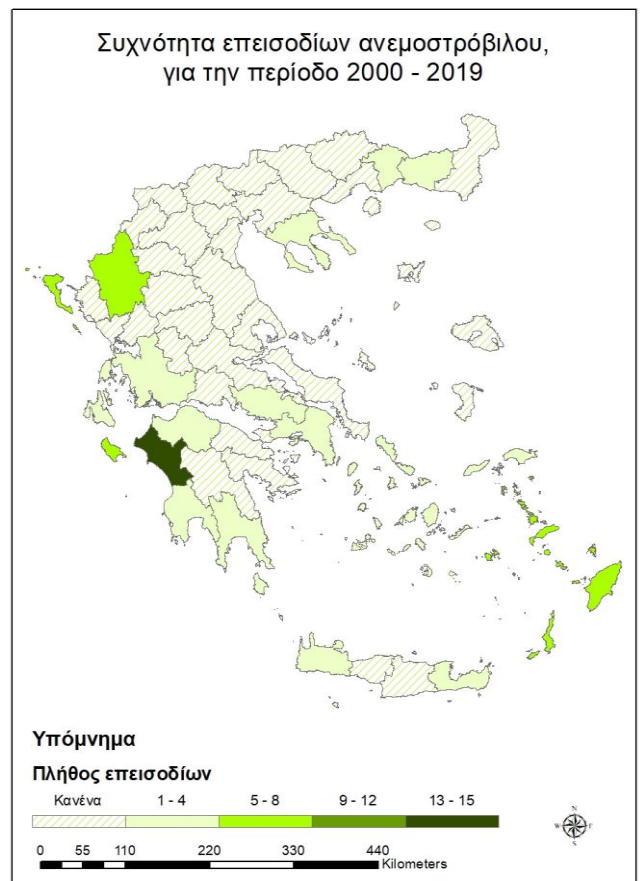
Σχήμα 16. Συχνότητα επεισοδίων ανεμοστρόβιλου με κοινωνικές και οικονομικές επιπτώσεις ανά νομό, για την περίοδο 2000 – 2019.
