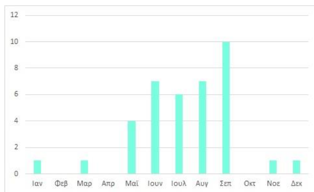
Σχήμα 5. Απώλειες ζωής από κεραυνικό πλήγμα, για την περίοδο 2000 - 2019
