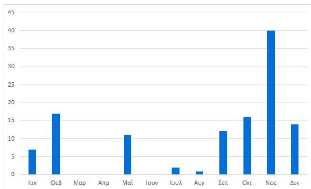
Σχήμα 7. Απώλειες ζωής από πλημμύρα για την περίοδο 2000 – 2019
