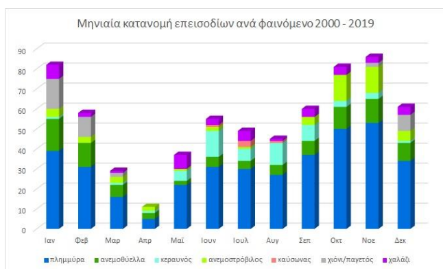
Σχήμα 9. Μηνιαία κατανομή επεισοδίων ανά φαινόμενο την περίοδο 2000 – 2019.
