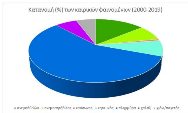
Σχήμα 8. Κατανομή (%) των καιρικών φαινομένων (2000 - 2019)
