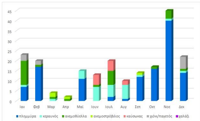
Σχήμα 6. Απώλειες ζωής ανά μήνα και καιρικό φαινόμενο, για την περίοδο 2000 – 2019
